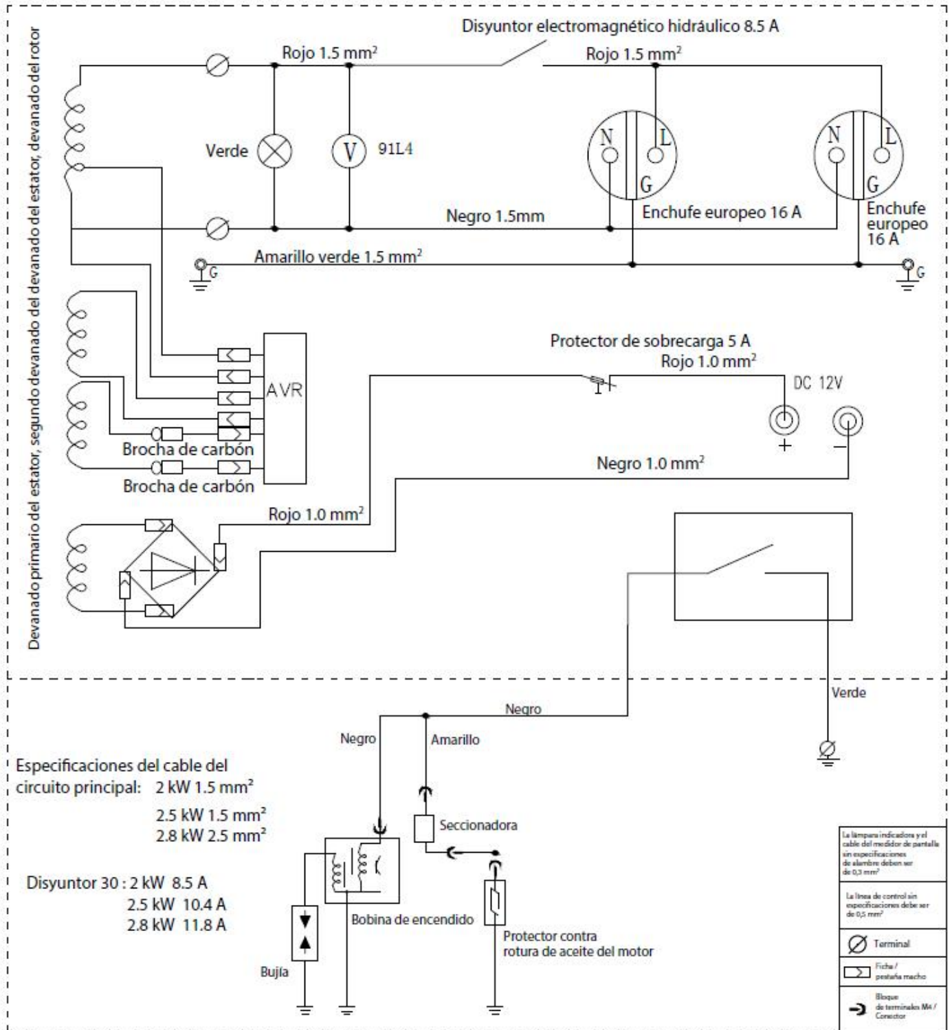
Diagrama Eléctrico Esquemá
